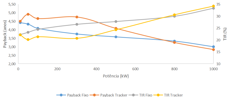
Figura 16 – Relação entre o payback e a TIR de sistemas fotovoltaicos fixos e com rastreamento de um eixo em função da potência instalada, para Belo Horizonte–MG.
