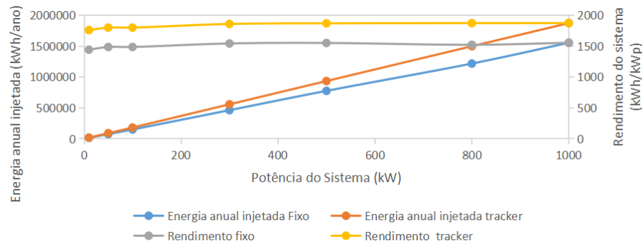
Figura 12 – Relação entre energia anual injetada e rendimento específico para sistemas fotovoltaicos com estrutura fixa e com rastreamento solar de um eixo em Belo Horizonte–MG.
