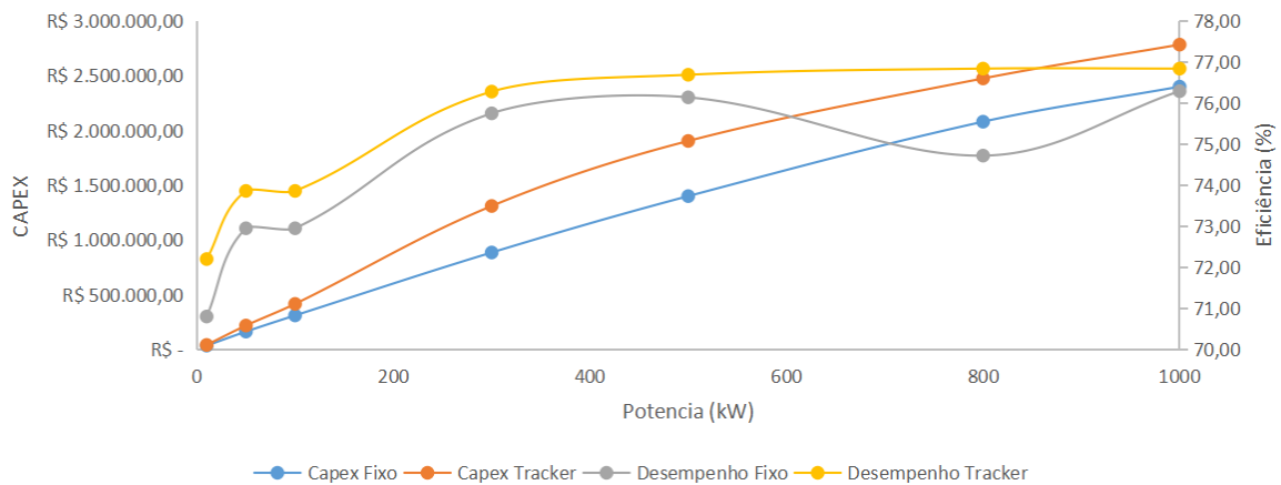
Figura 14 – Relação entre o investimento inicial (CAPEX) e a eficiência global de sistemas fotovoltaicos de estrutura fixa e com rastreamento solar de um eixo, em função da potência instalada, para as condições de Belo Horizonte–MG.
