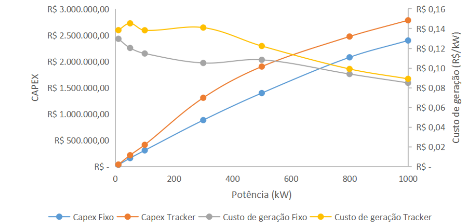
Figura 15 – Relação entre o CAPEX e o custo de geração de energia (R$/kWh) de sistemas fotovoltaicos fixos e com rastreamento de um eixo em função da potência instalada, para Belo Horizonte–MG.
