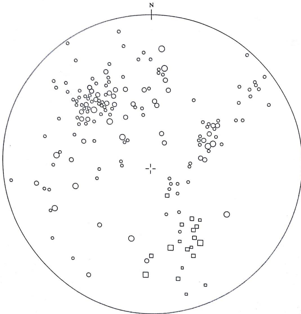
Figura 3.8 - Exemplo de aglomeração de polos. Fonte: adaptado de PRIEST (1985).
